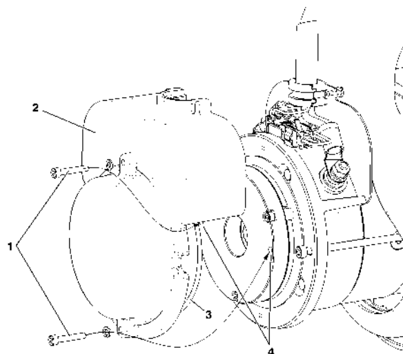
Figura 4-3. Desenganche manual
