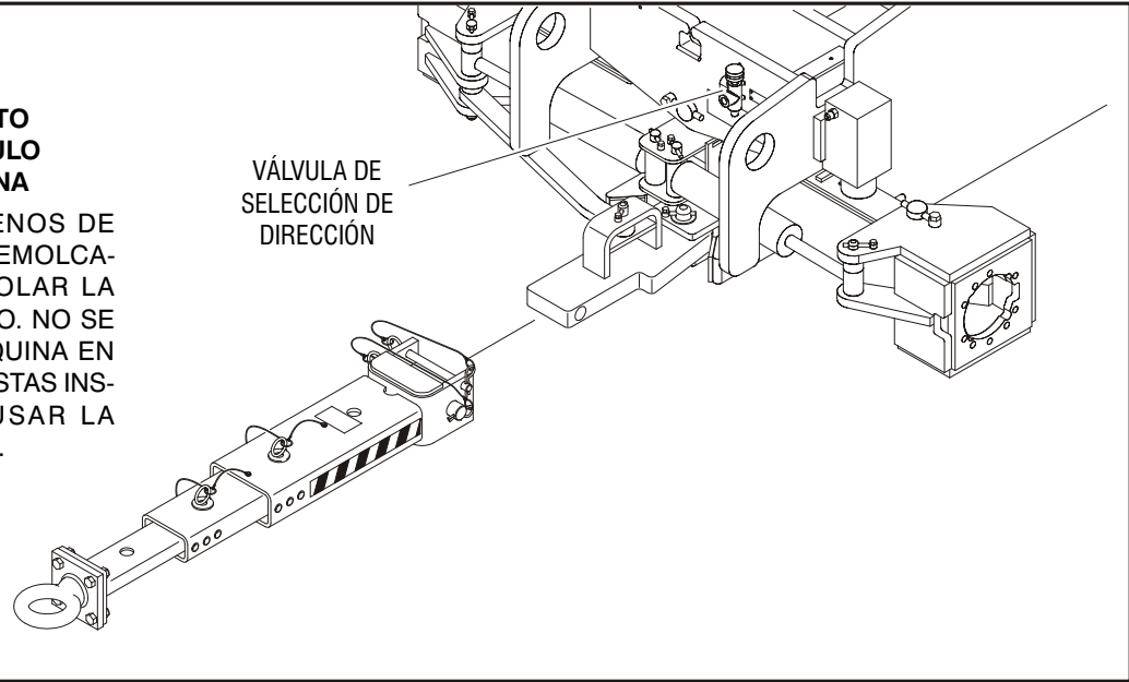
Figura 4-6. Puntos de conexión de barra de remolcado - Máquinas con NS 75606 al presente
