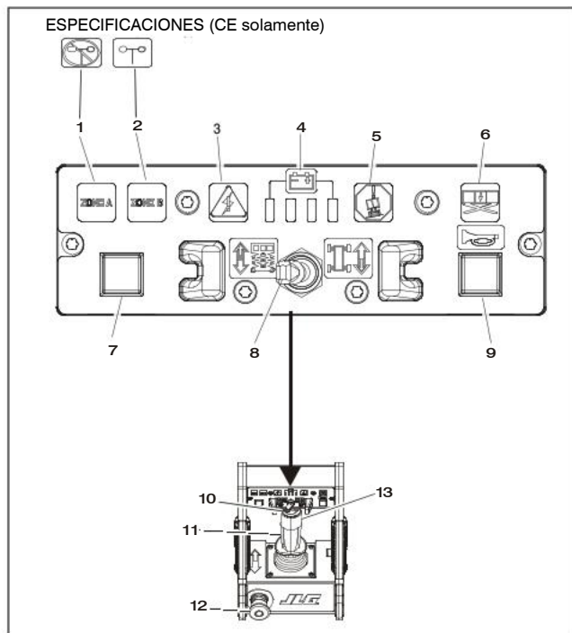
Figura 3-3. Puesto de controles de plataforma
