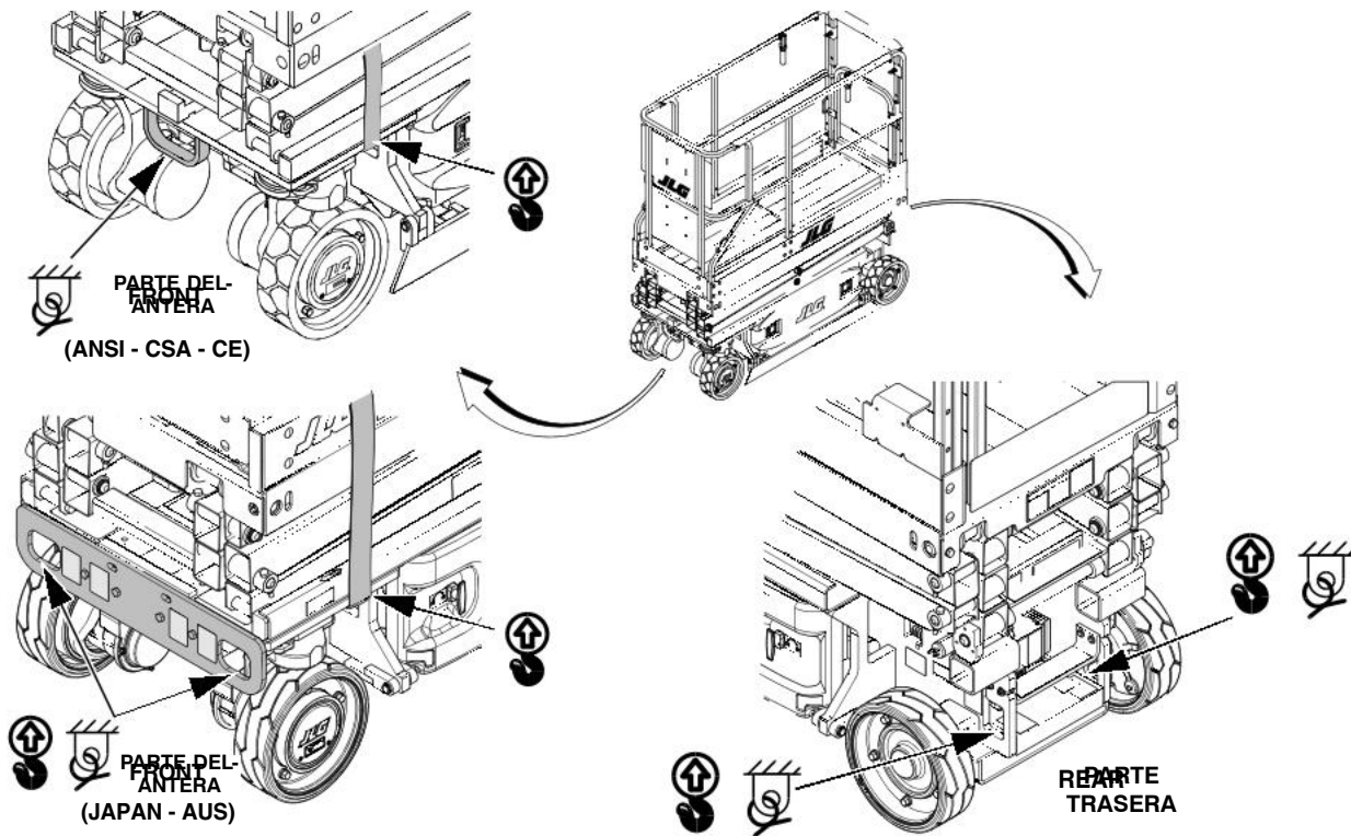
Figura 4-2. Diagrama de levante y amarre
