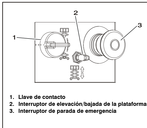
Figura 3-1. Puesto de controles de suelo
