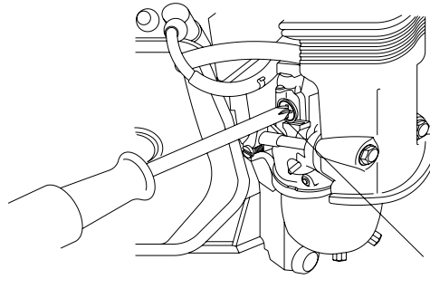
2. Tornillo de tope de mariposa
